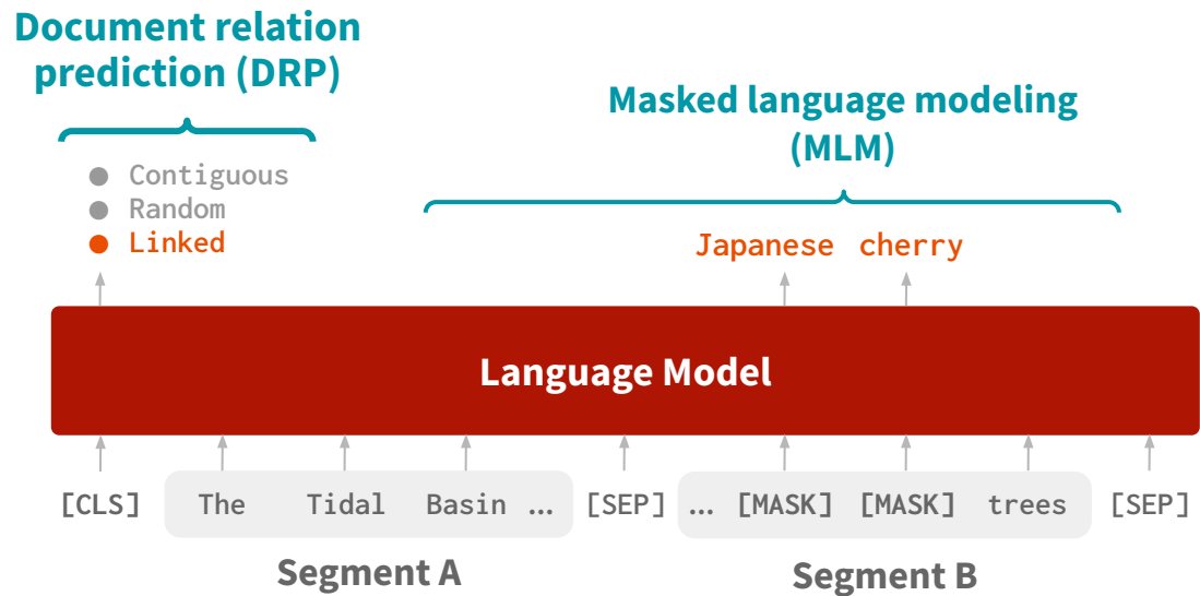
Pretrain the LM
